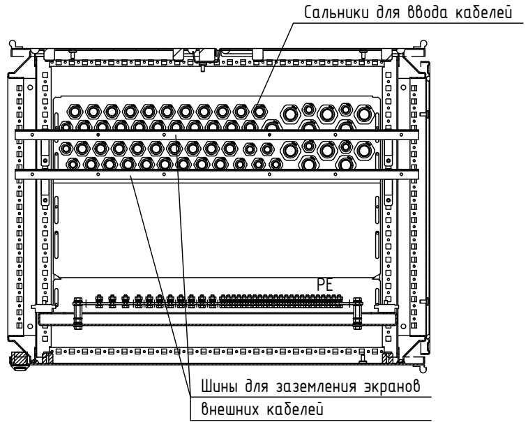
Б-Б
